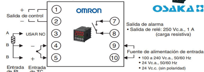
Omron E5CB
